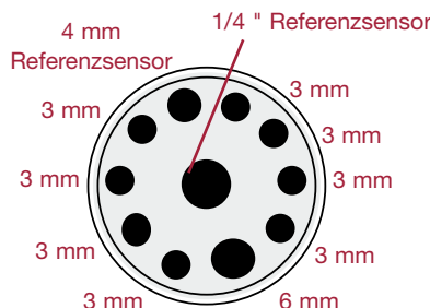
Mehrfachbohrung M03 (ATC-125 A/B)
