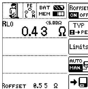
Menü Niederohmmessung
