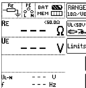
Menü Erdwiderstandsmessung
