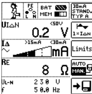
Menü RCD-Messung
