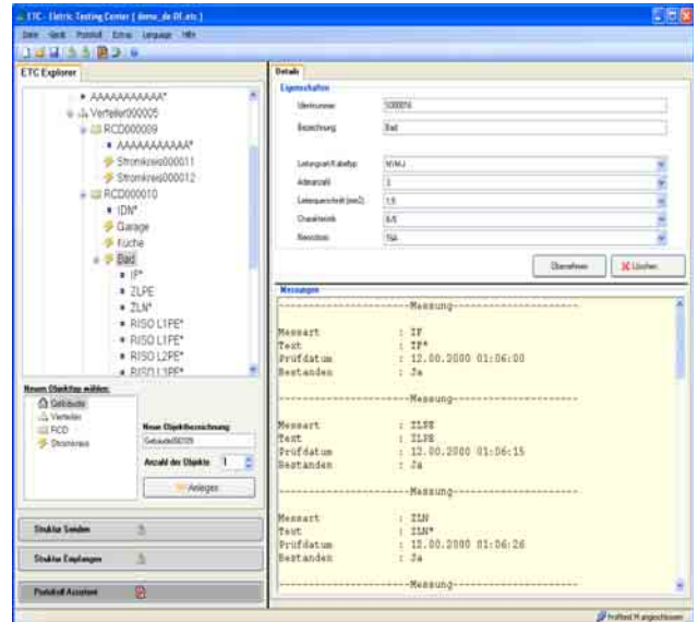
Menü Schleifenwiderstandsmessung
