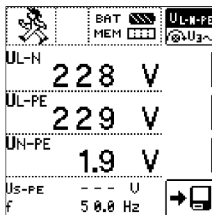
Menü Spannungsmessung
