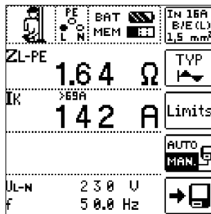
Menü Schleifenwiderstandsmessung
