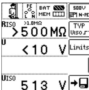
Menü Isolationsmessung
